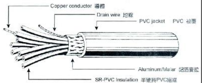
單層芯型鋁箔麥拉整體隔離電腦信號電纜
